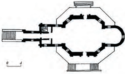
106. Володимирсько-Богородична церква. Вул. Осіння, 12. Схематичний план, 1984.
