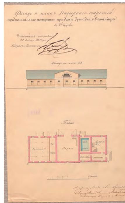
1.1. План і фасад надвірної будівлі, 1835.
