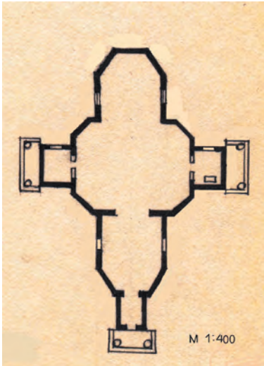
19. Церква Введенська, смт Введенка, вул. Озерна, 19. План церкви.
