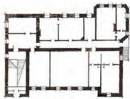
19. Вул. Старонікольська, 35. Схематичний план 1-го поверху.
