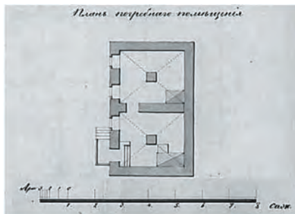
1.5. План цокольного поверху.
