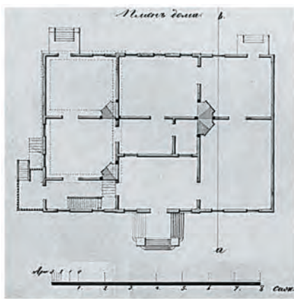
1.5. Пл. Соборна, 2-а. План будинку.
