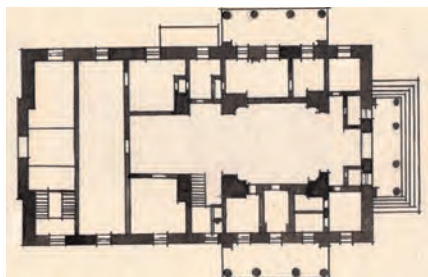
1.3. Вул. Фортешний узвіз, 5. Схематичний план будівлі (з 1984 до 2010).
