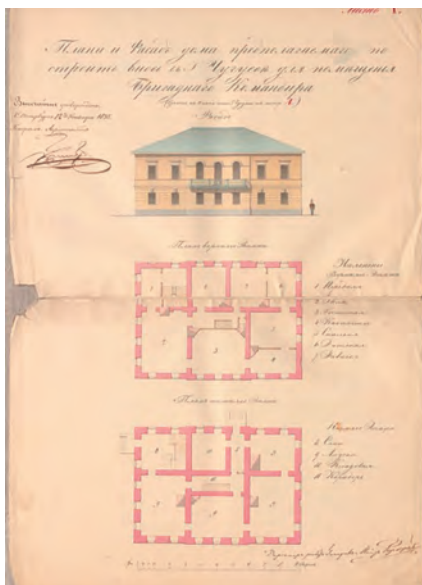
1.1. План і фасад будинку бригадного командира, 1838.
