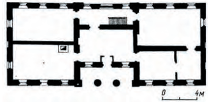
97. План 1-го поверху кол. корпусу ескадронного комітету (північного корпусу), 1984.
