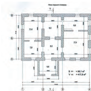
5. Вул. Музейна, 8. План першого поверху до реставрації.
