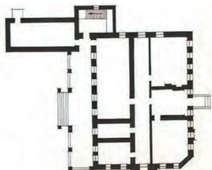
7.7. Вул. Гвардійська, 52. Схематичний план 1-го поверху.
