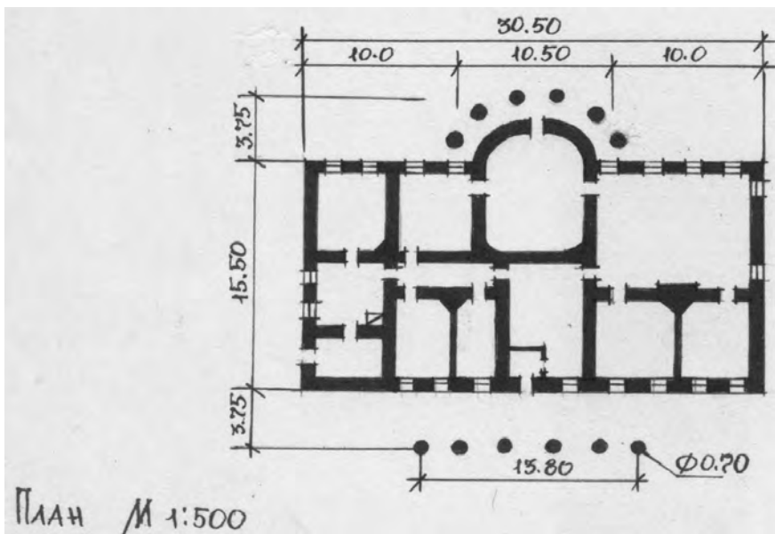
130. План будівлі.
