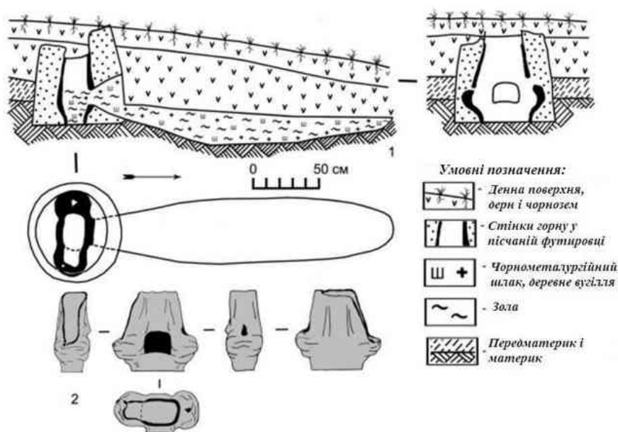
20. Схема чорнометалургійного горна-В з ремісничого центру «Уроцище Роганіна» та малюнок його колби-тигля.
