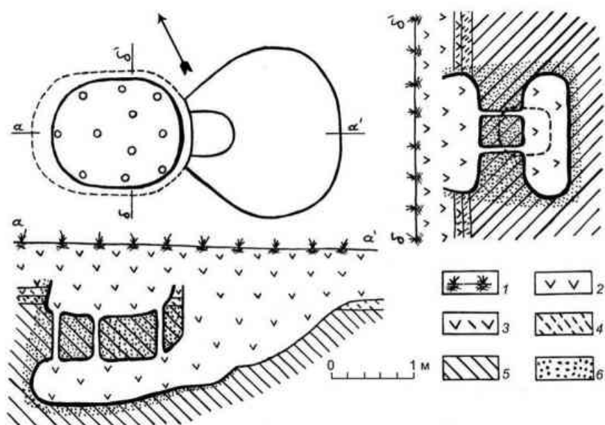
20. Схема гончарного горна-А з ремісничого центру «Уроцище Роганіна». Умовні позначення: 1 — дерен, 2 — чорнозем, 3 — давній ґрунт, 4 — передматерик, 5 — материк, 6 — зона пропеченого ґрунту.
